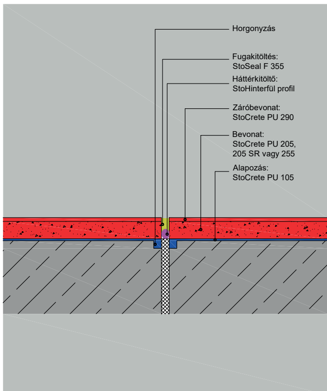
Csomópont 3: dilatáció tömítése
