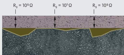
A kiegyenlítő glettelés biztosítja a felső réteg egyenletes rétegvastagságát és ezáltal az egyenletes ellenállást
